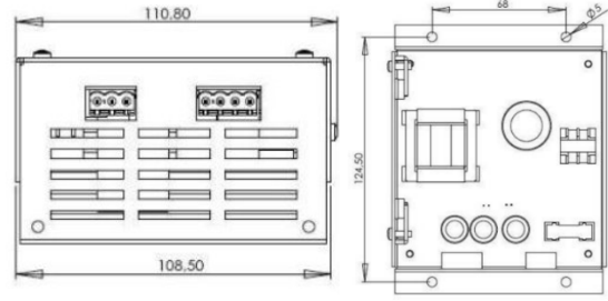
Resim 2: Boyutlar mm cinsinden gösterilmiştir.
