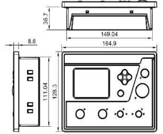
Resim 2: AMF-M Boyutlar (mm)
